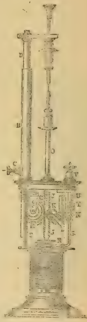
1 מנורת דיפרנציאלית
